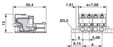
Rysunek wymiarowy
