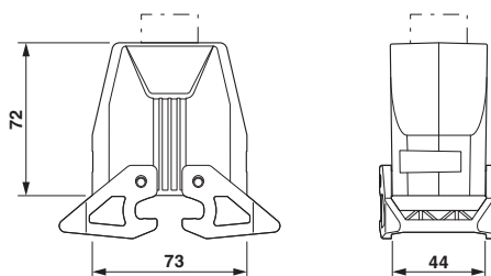
Rysunek wymiarowy
