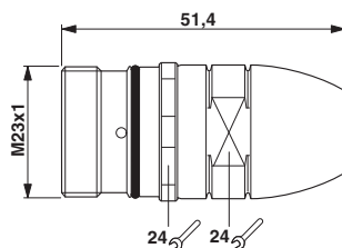
Rysunek wymiarowy
