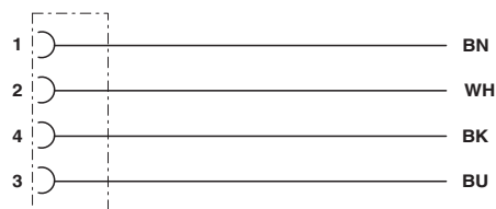
Przyporządkowanie styków wtyków / gniazdz M8 / M12
