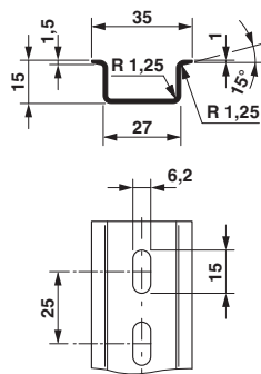
Rysunek wymiarowy
