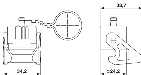
Rysunek wymiarowy
