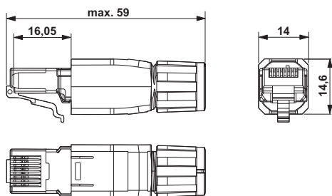
Rysunek wymiarowy
