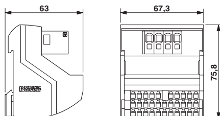
Rysunek wymiarowy
