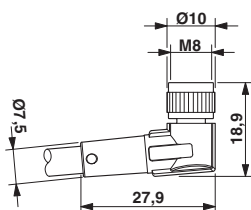
Rysunek wymiarowy
