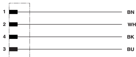
Przyporządkowanie styków wtyku M8
