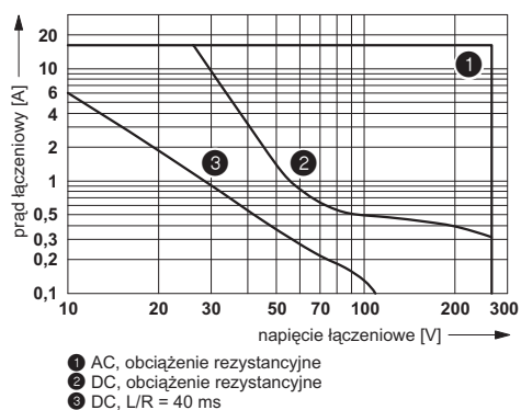
Zdolność wyłączenia
