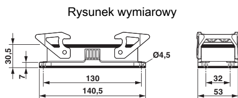
Rysunek wymiarowy
