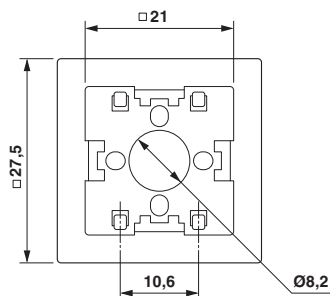
Rysunek wymiarowy
