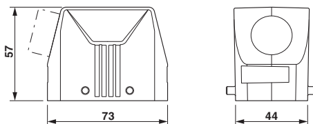
Rysunek wymiarowy
