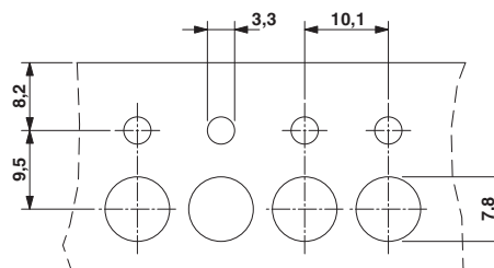
Rysunek wymiarowy
