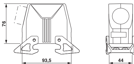
Rysunek wymiarowy
