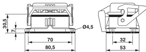
Rysunek wymiarowy
