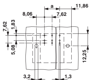
Szablon wierceń
