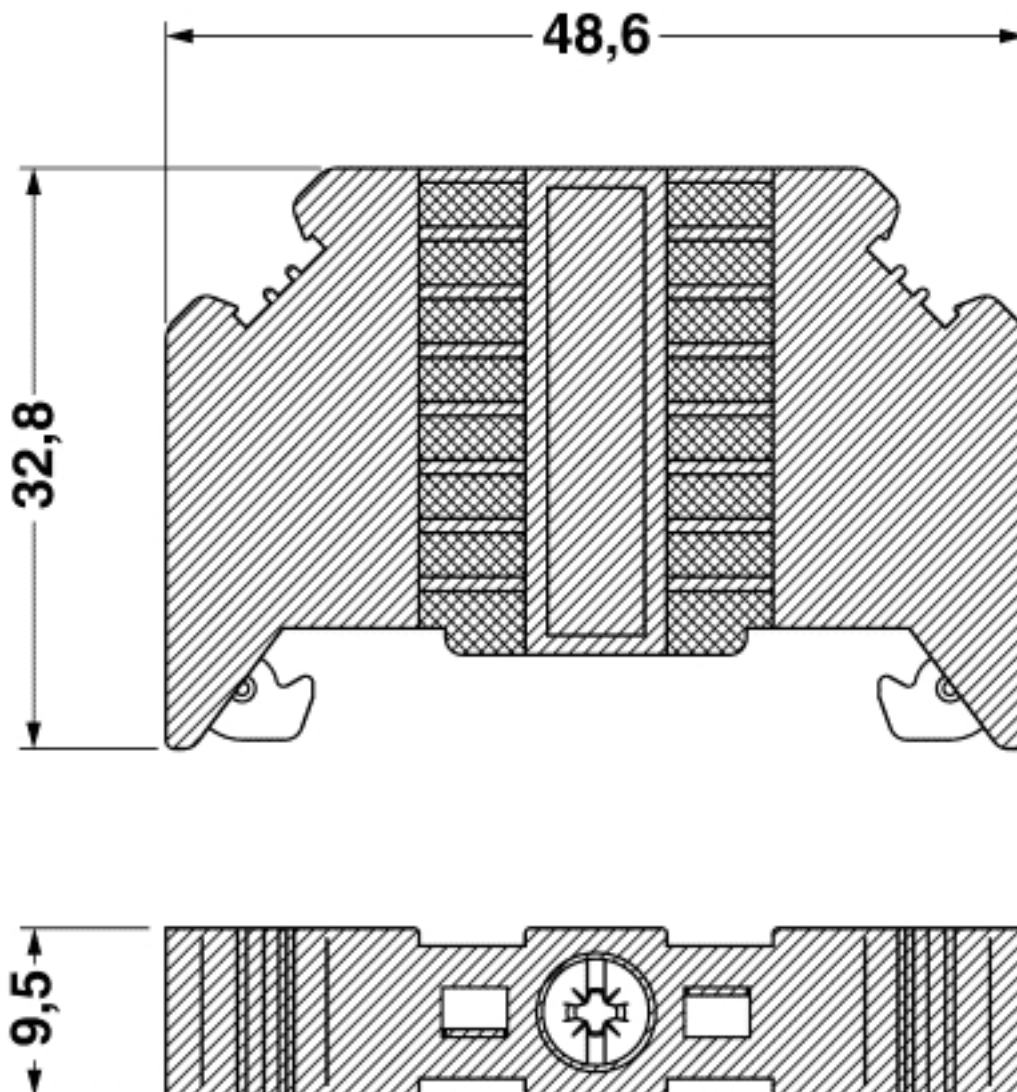
Rysunek wymiarowy
