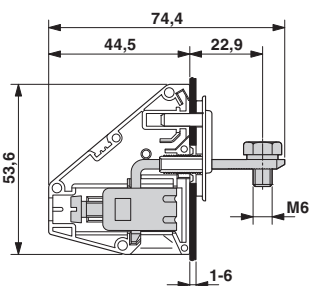
Rysunek wymiarowy
