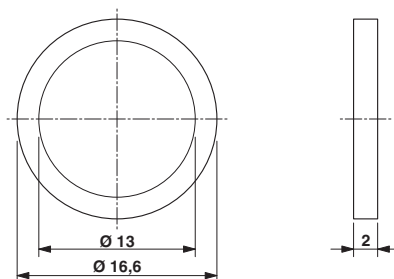
Rysunek wymiarowy
