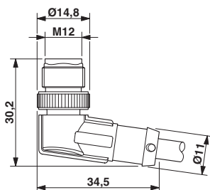
Rysunek wymiarowy
