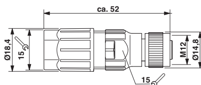
Rysunek wymiarowy
