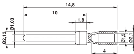
Rysunek wymiarowy
