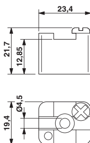
Rysunek wymiarowy
