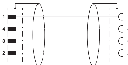
Przyporządkowanie styków wtyków M12 i gniazd M12
