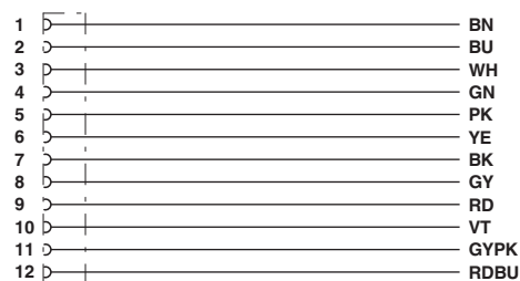
Przyporządkowanie styków gniazda M12
