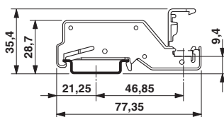
Rysunek wymiarowy
