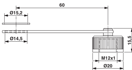
Rysunek wymiarowy
