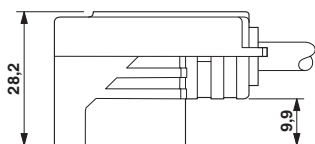
Wtyk zaworowy, typ BI, widok z boku
