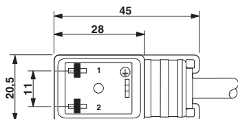
Wtyk zaworowy typ BI
