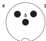
Układ styków wtyk M12, 3-biegunowy, wtyk zaworowy
