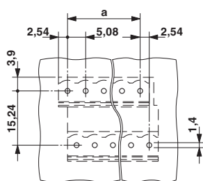
Szablon wierceń
