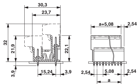
Rysunek wymiarowy
