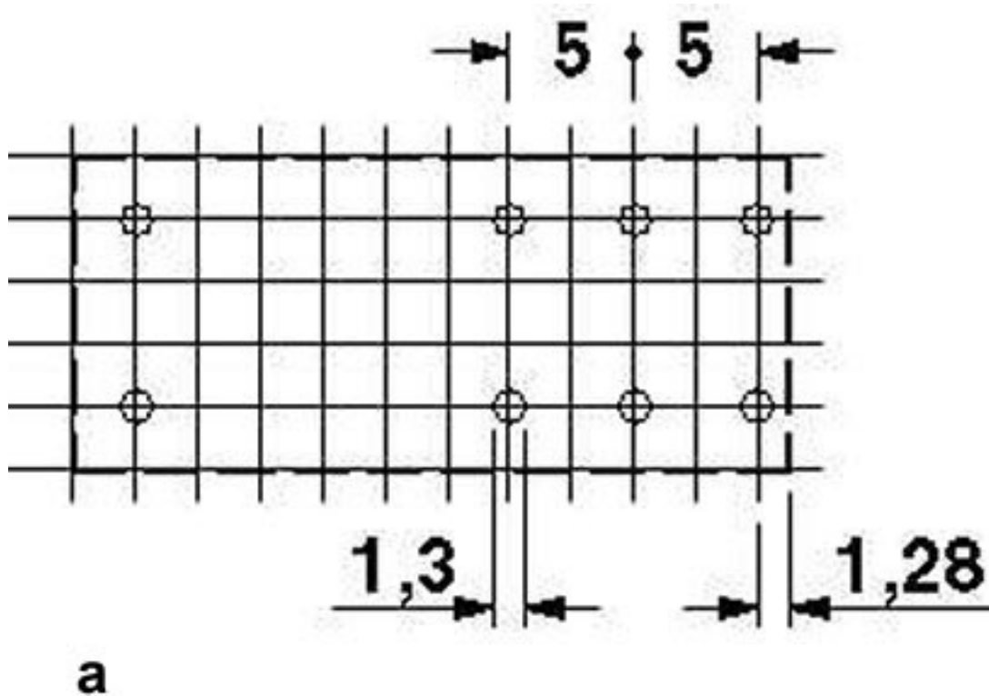
Szablon wierceń
