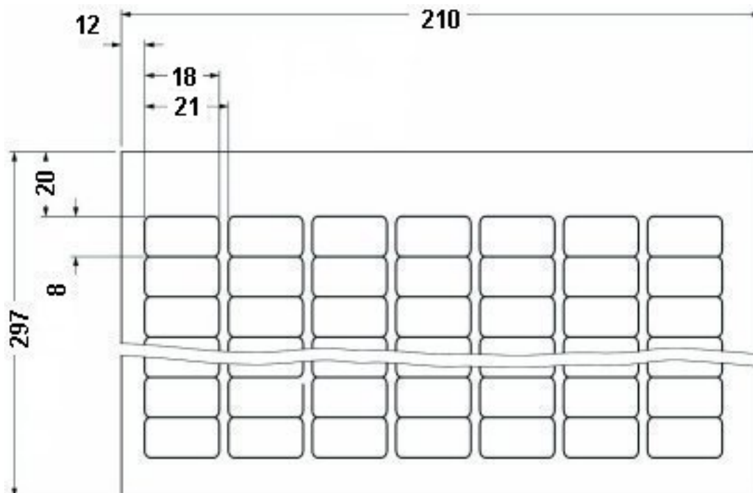
Rysunek wymiarowy
