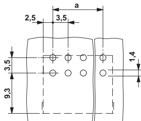
Szablon wierceń
