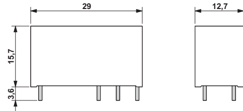
Rysunek wymiarowy
