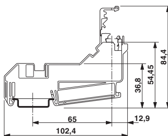
Rysunek wymiarowy
