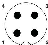
Układ styków, wtyk M12, 4-biegunowy, kodowanie A, widok od strony styków męskich
