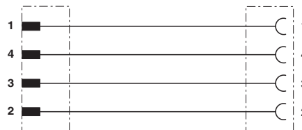
Przyporządkowanie styków wtyków M12 / gniazda M8
