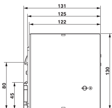
Rysunek wymiarowy
