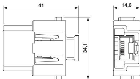
Moduł wkładki stykowej
