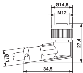
Rysunek wymiarowy
