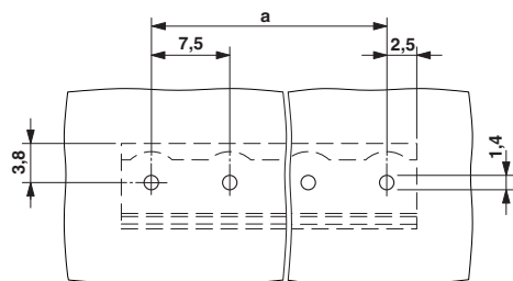
Szablon wierceń
