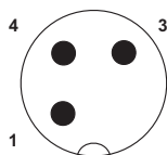
Układ biegunów wtyku męskiego M12, 3-biegunowy, z kodowaniem typu A, widok od strony z kółkami
