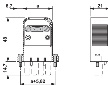
Rysunek wymiarowy
