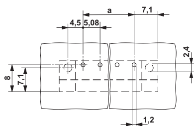
Szablon wierceń
