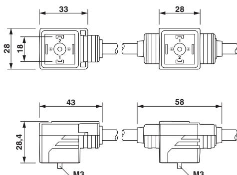
Podwójny wtyk zaworowy, 2x konstrukcja A
