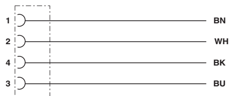
Przyporządkowanie styków gniazda M12
