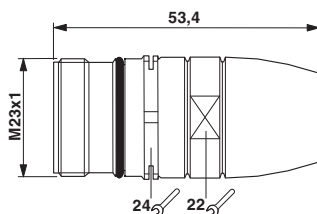
Rysunek wymiarowy
