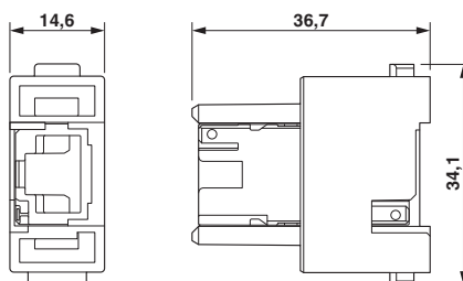
Rysunek wymiarowy
