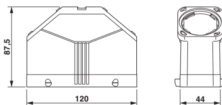
Rysunek wymiarowy
