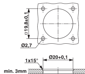
Rysunek wymiarowy
